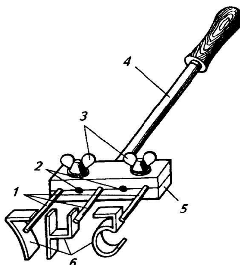
Рис. 18. Приспособление для термального мечения рыб: 1-штоки; 2-отверстия для закрепления матриц; 3- винты; 4- рукоятка; 5 - державка; 6- матрицы
